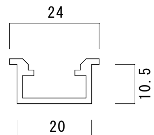
レールの詳細（HD-01）
